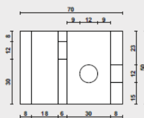
SEZIONE
